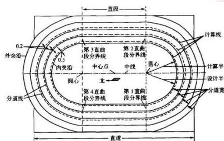
图 7-1 半圆式田径场的结构 (单位:m)
